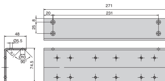
Угловая монтажная пластина 7103
